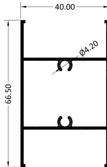
3653 TRAVESAÑO 66.50 MM
