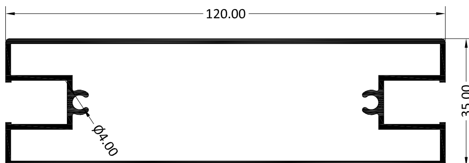
3654 TRAVESAÑO 120 MM
