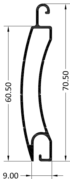
4520 LAMA DE PERSIANA DE 60
