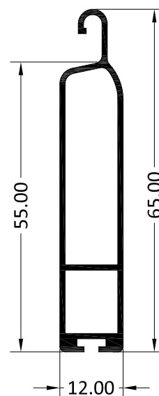
4521 TERMINAL DE PERSIANA DE 55
