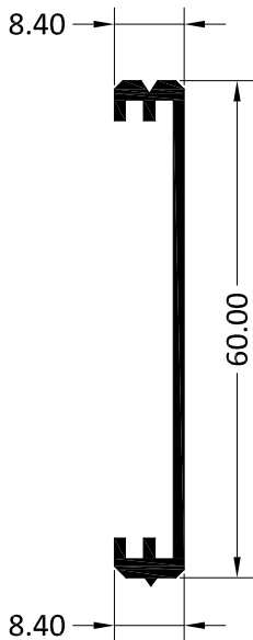
10018 LAMA DE FORRO 60
