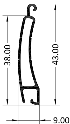
4519 LAMA DE PERSIANA DE 38
