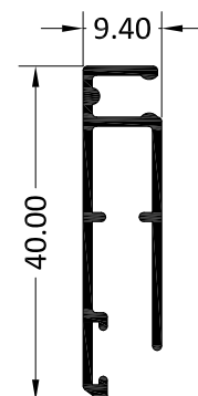
4201 PERFIL MOSQUITERA DE 40
