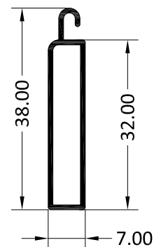
4522 TERMINAL DE PERSIANA DE 32
