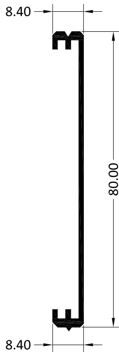
10017 LAMA DE FORRO 80
