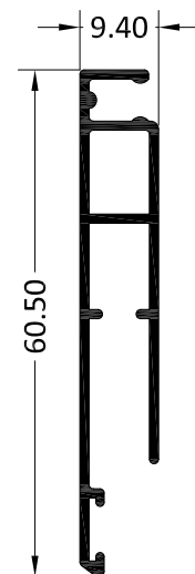
4200 PERFIL MOSQUITERA DE 60.50
