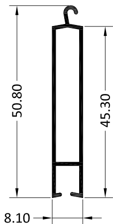
4523 TERMINAL DE PERSIANA DE 51
