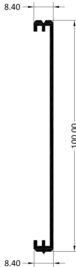
10016 LAMA DE FORRO 100
