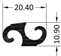
4560 UNIÓN ENTRE LAMAS
